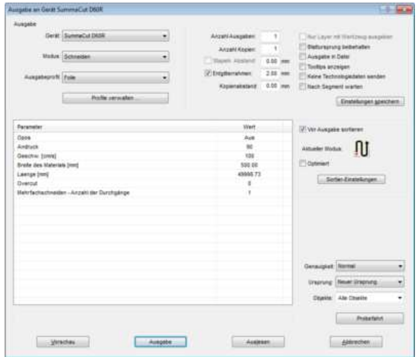
Ausgabefenster - Treiberauswahl und Schneideparameter-Setup
